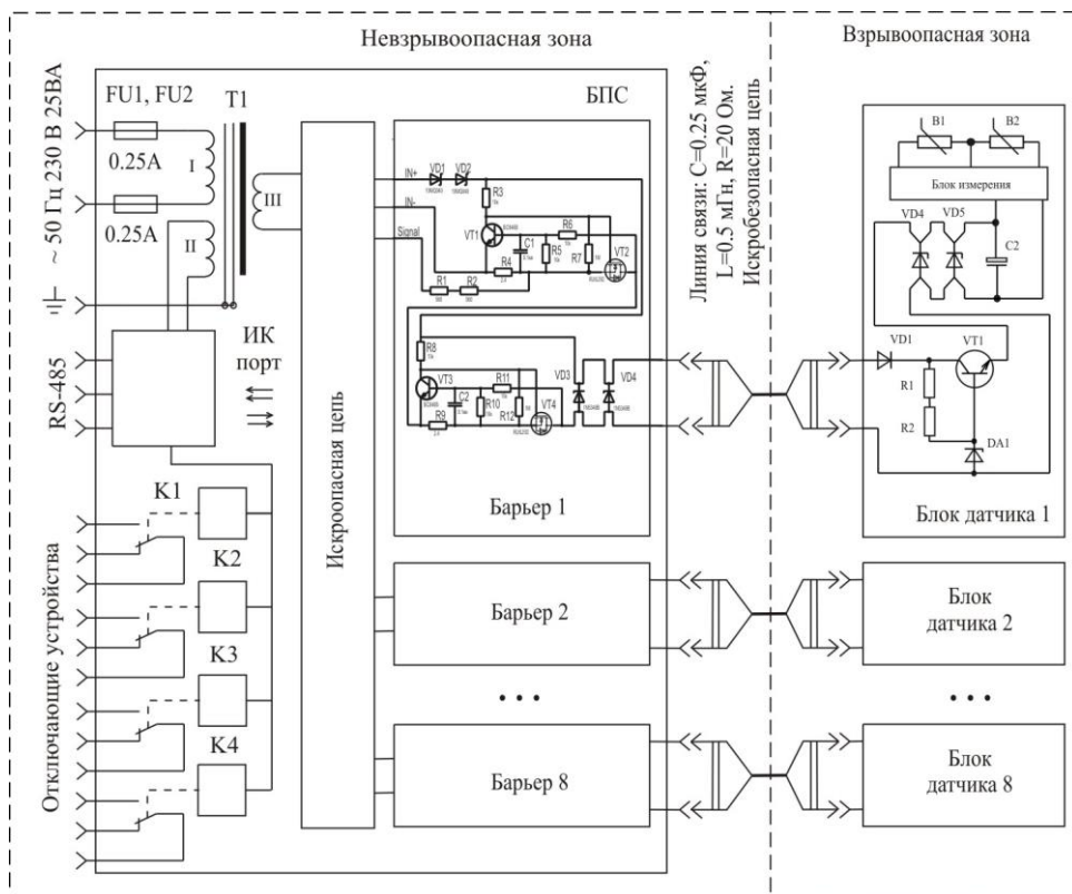
Рисунок 5.1 Средства обеспечения взрывозащитности БПС 230В
