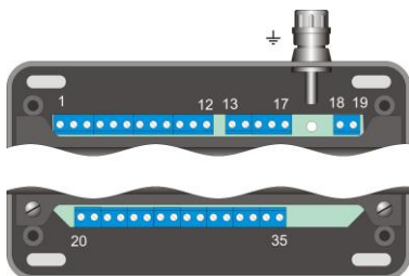
Рисунок 6.2 Клеммы БПС 230В.
