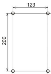
Рисунок 6.1. Разметка для крепления
