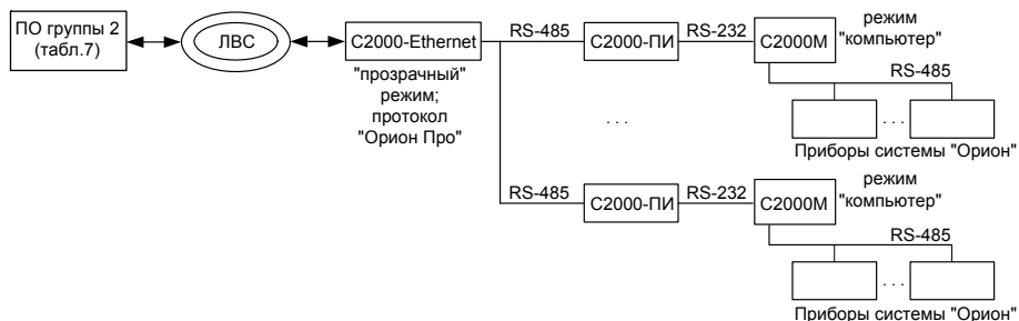
Рисунок 4 Схема подключения нескольких пультов «C2000»/«C2000М» к одному виртуальному СОМ-порту
