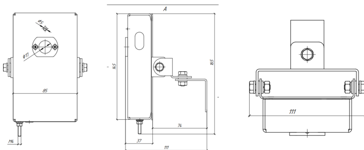
Рисунок А2 – Габаритные размеры Спектрон-801-М, -801-Н, -801-Ехі-М, -801-Ехі-Н, -801-Ехм-М, -801-Ехм-Н
