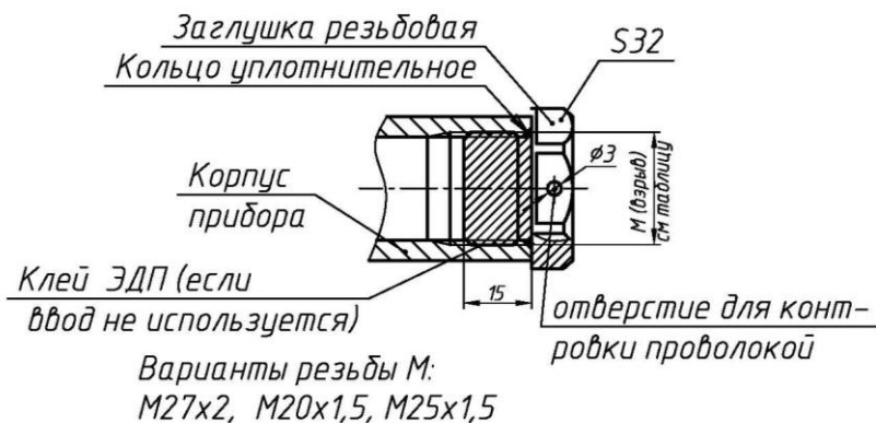
Рисунок А.3 – Элементы взрывозащиты при поставке извещателя с резьбовыми заглушками
