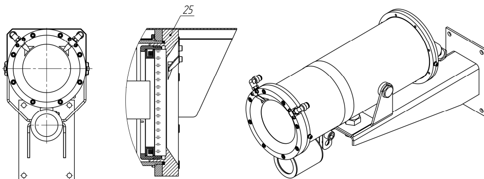
Рисунок 5. Внешний вид термокожуха ТВК-07-Н/С с установленным фланцем (СОД) для работы с системой очистки стекла “Дуплекс-07с”-Ех-ТВК-Х.
