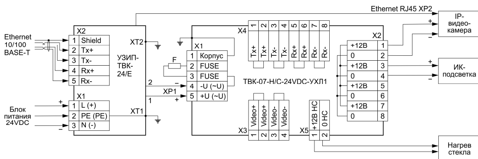
г) Подключение термокожуха на примере модификации ТВК-07-С-24VDC-УХЛ1 с устройством защиты УЗИП-ТВК-24/Е и IP-видеокамерой
