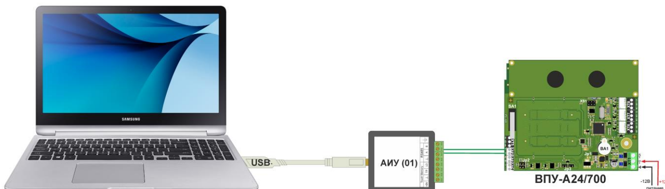
Рисунок 93. Схема подключения для программирования ВПУ-A24/700
