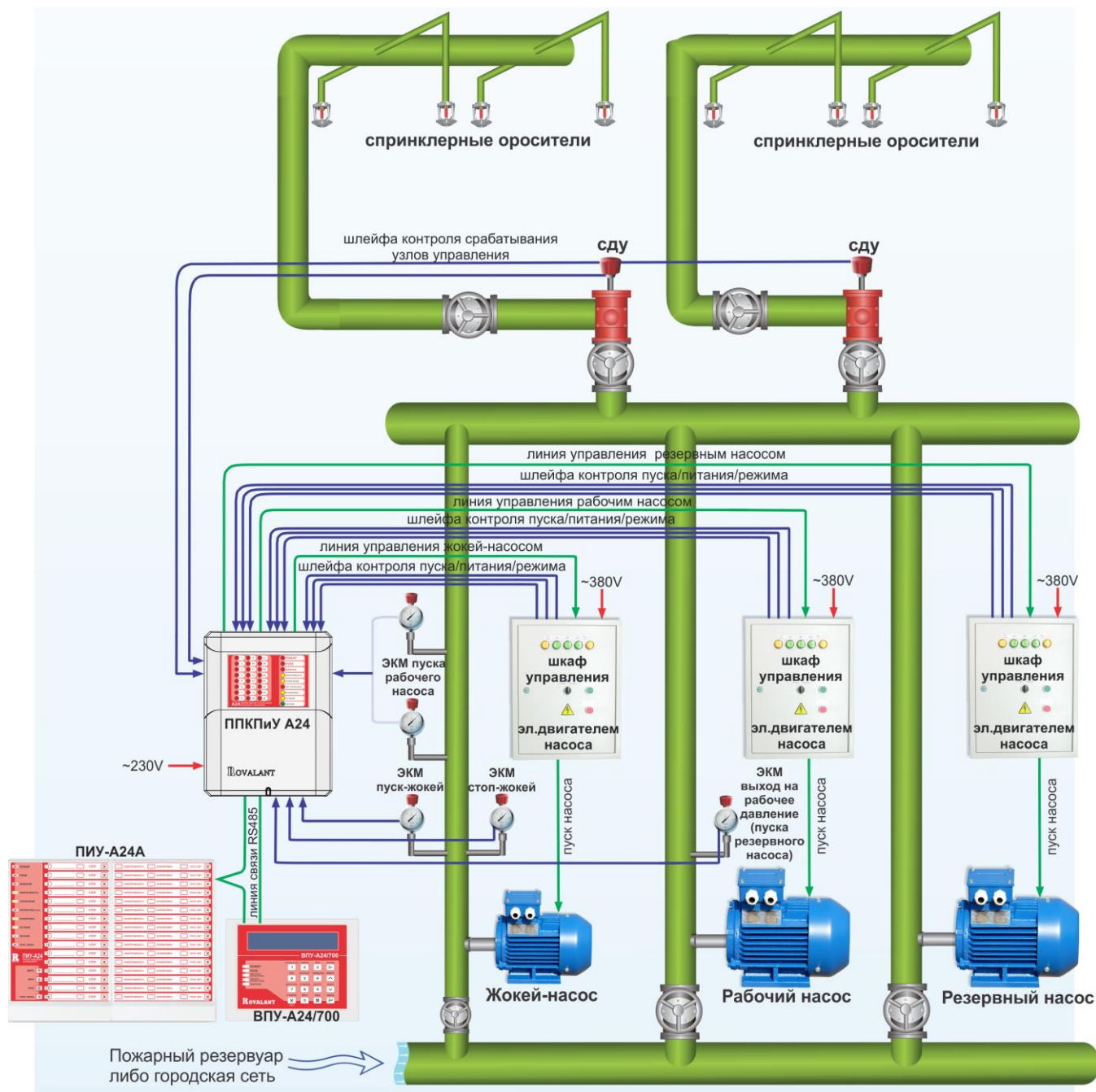
Рисунок 97. Пример автоматизации спринклерной установки водозаполненной системы водяного АПТ.
