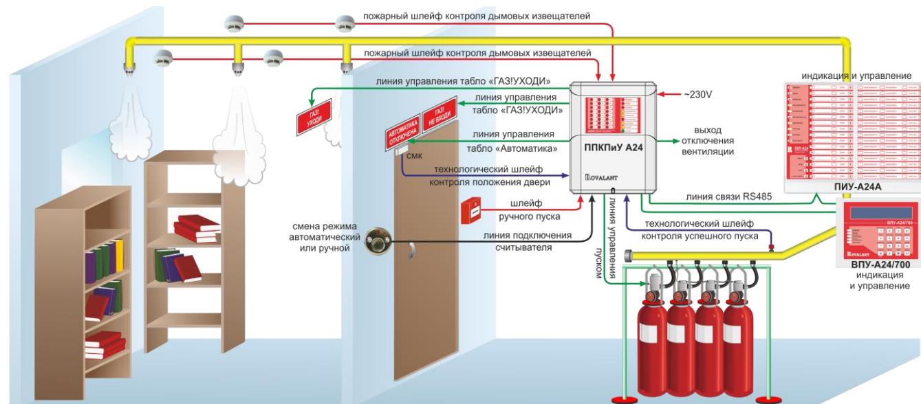
Рисунок 95. Пример автоматизации системы модульного газового АПТ
