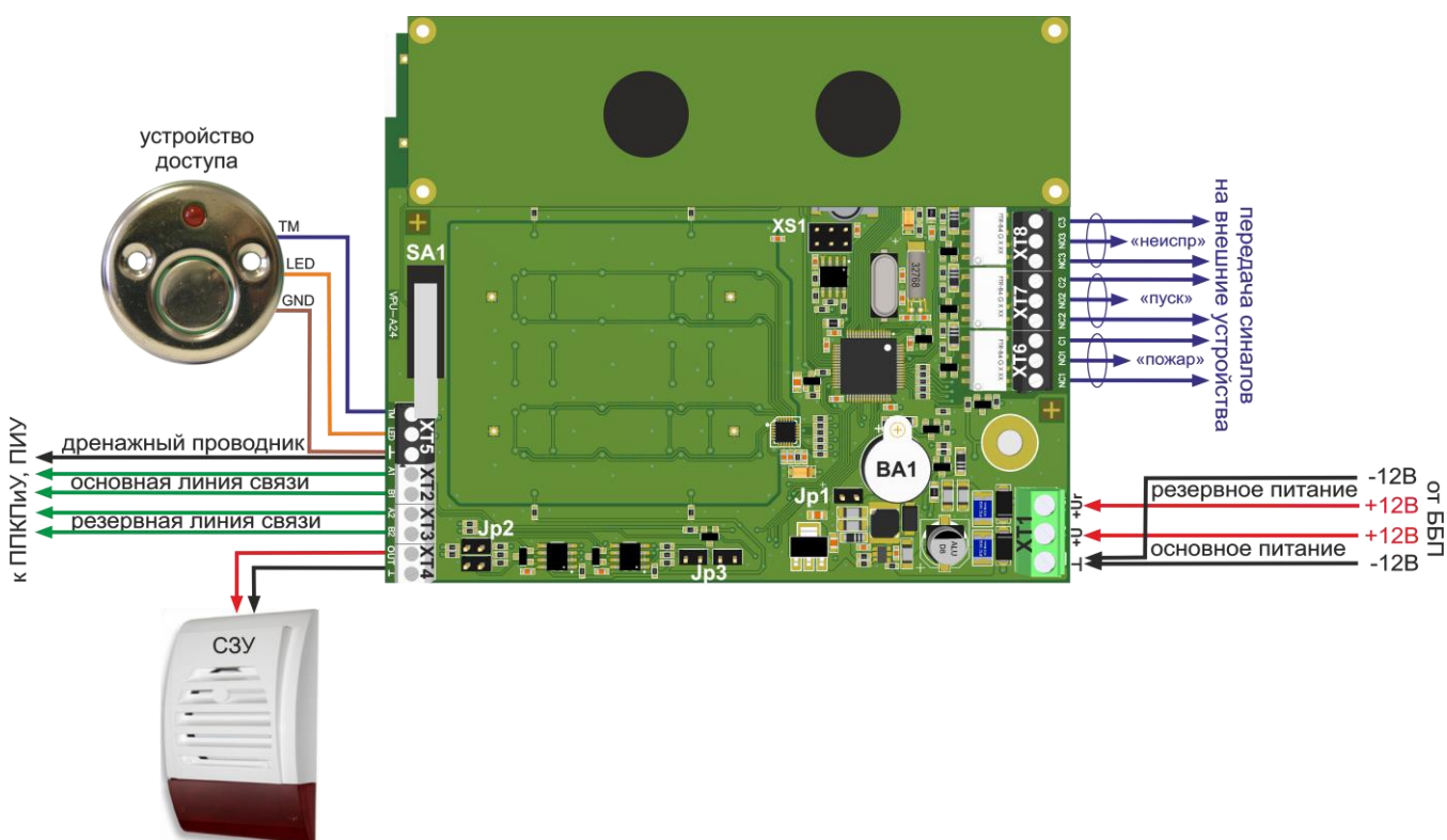
Рисунок 15. Схема подключения ВПУ-А24/700
