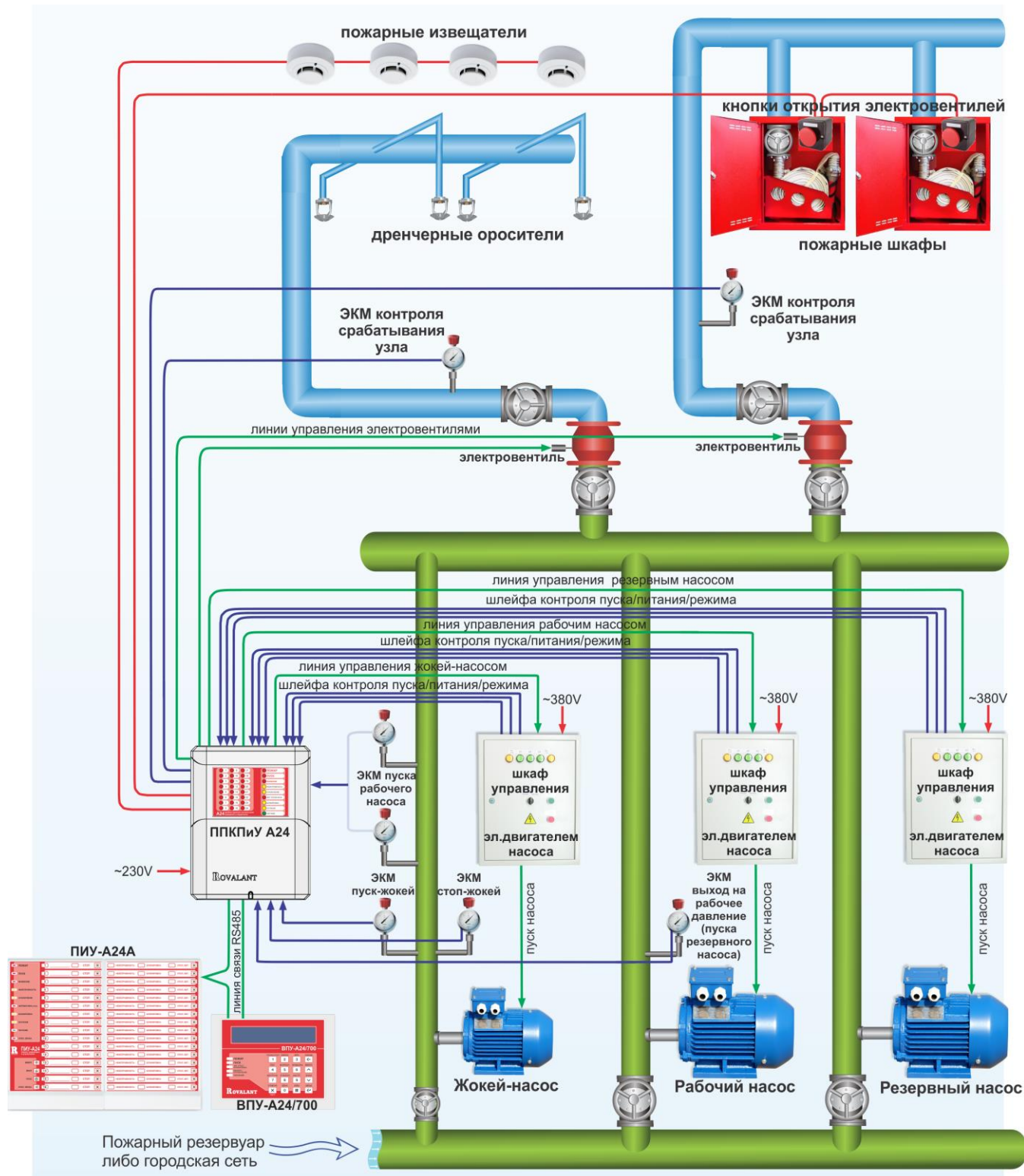
Рисунок 99. Пример автоматизации дренажной установки системы водяного АПТ.
