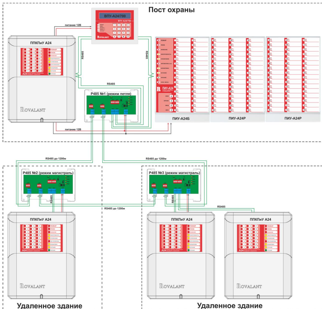
Рисунок 75. Схема подключения P485 для организации кольцевой гальвано-развязанной линии связи с сегментированной защитой от коротких замыканий.
