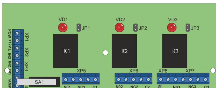
Рисунок 81. Внешний вид платы и обозначение элементов БУНЗ-12
