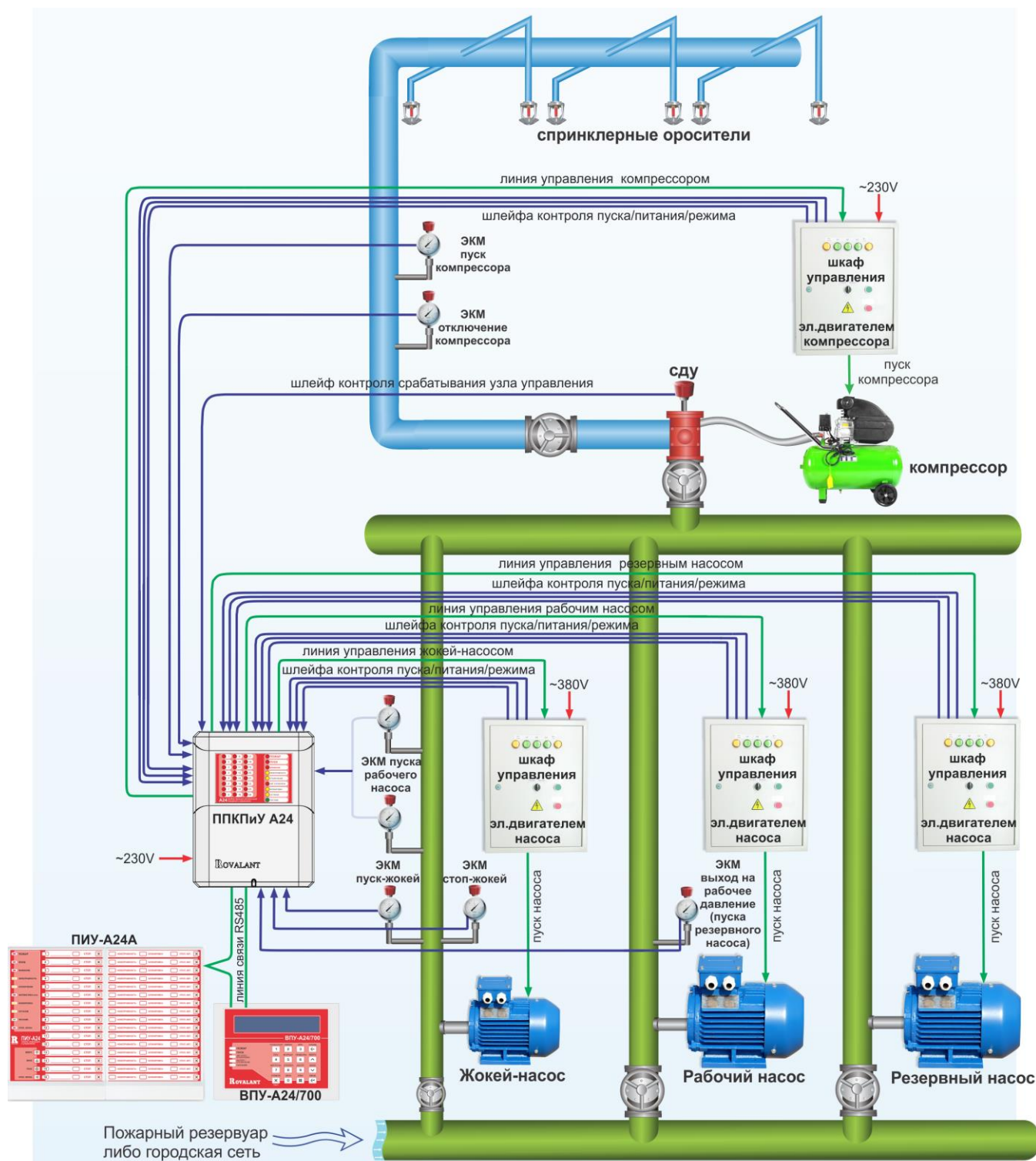
Рисунок 98. Пример автоматизации спринклерной установки воздухозаполненной системы водяного АПТ.
