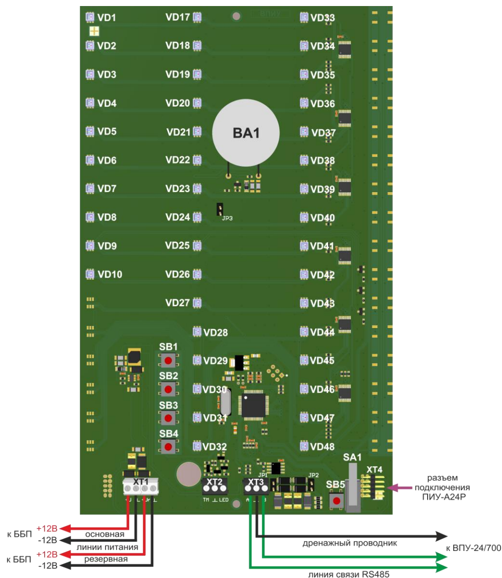
Рисунок 66. Внешний вид и подключение платы ПИУ-A24Б
