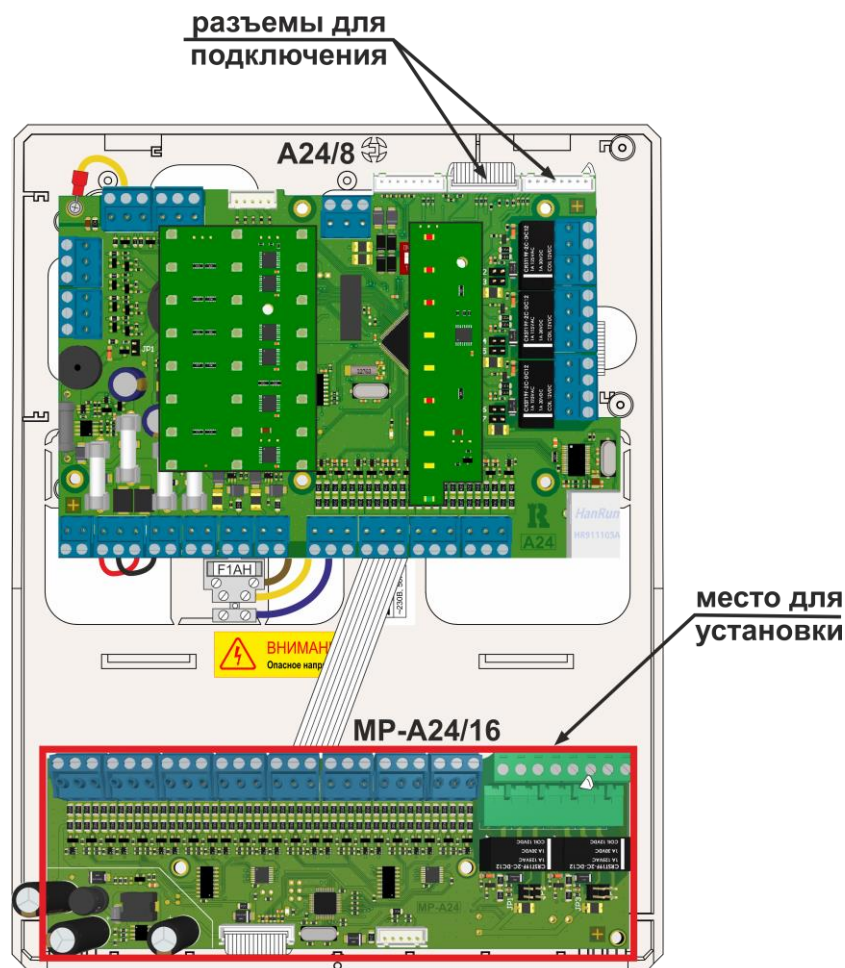
Рисунок 7. Установка и подключение MP-A24/16 к ППКПиУ
