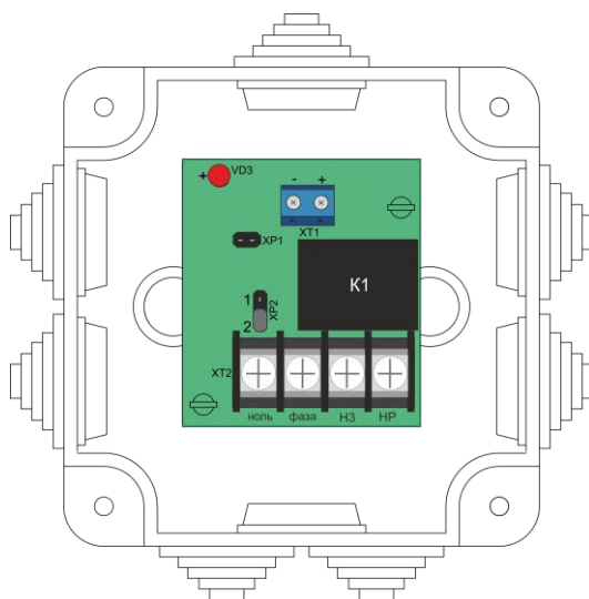
Рисунок 76. Внешний вид БУН1-12С (со снятой крышкой корпуса).
