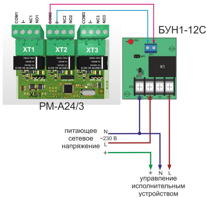
Рисунок 79. Схема подключения БУН1-12С к PM-A24/3.
