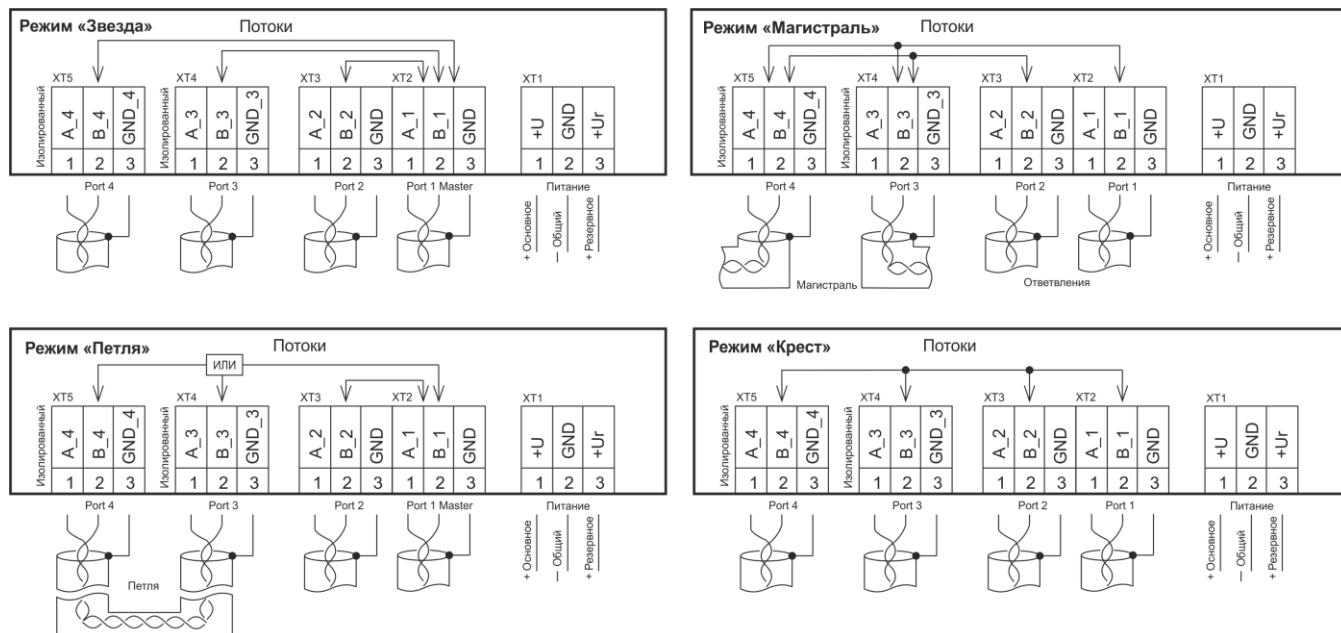
Рисунок 74. Подключение Р485 при различных режимах его работы
