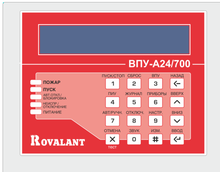
Рисунок 13. Внешний вид ВПУ-А24/700
