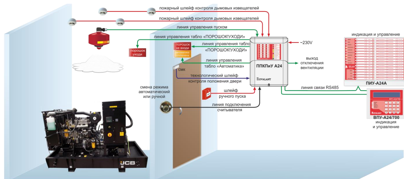
Рисунок 96. Пример автоматизации системы модульного порошкового АПТ
