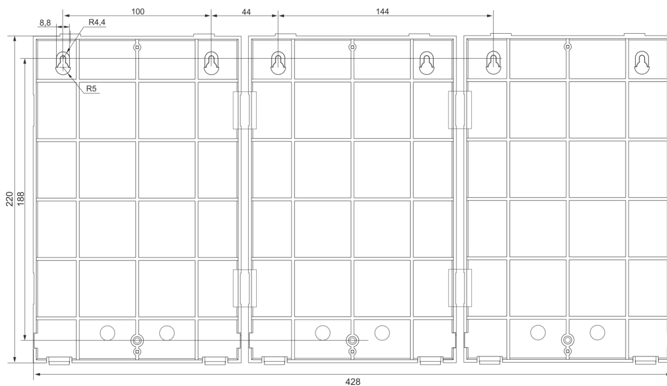
420 Рисунок 89. Установочный чертеж основания корпуса ПИУ-А24Б при применении совместно с двумя ПИУ-А24Р
