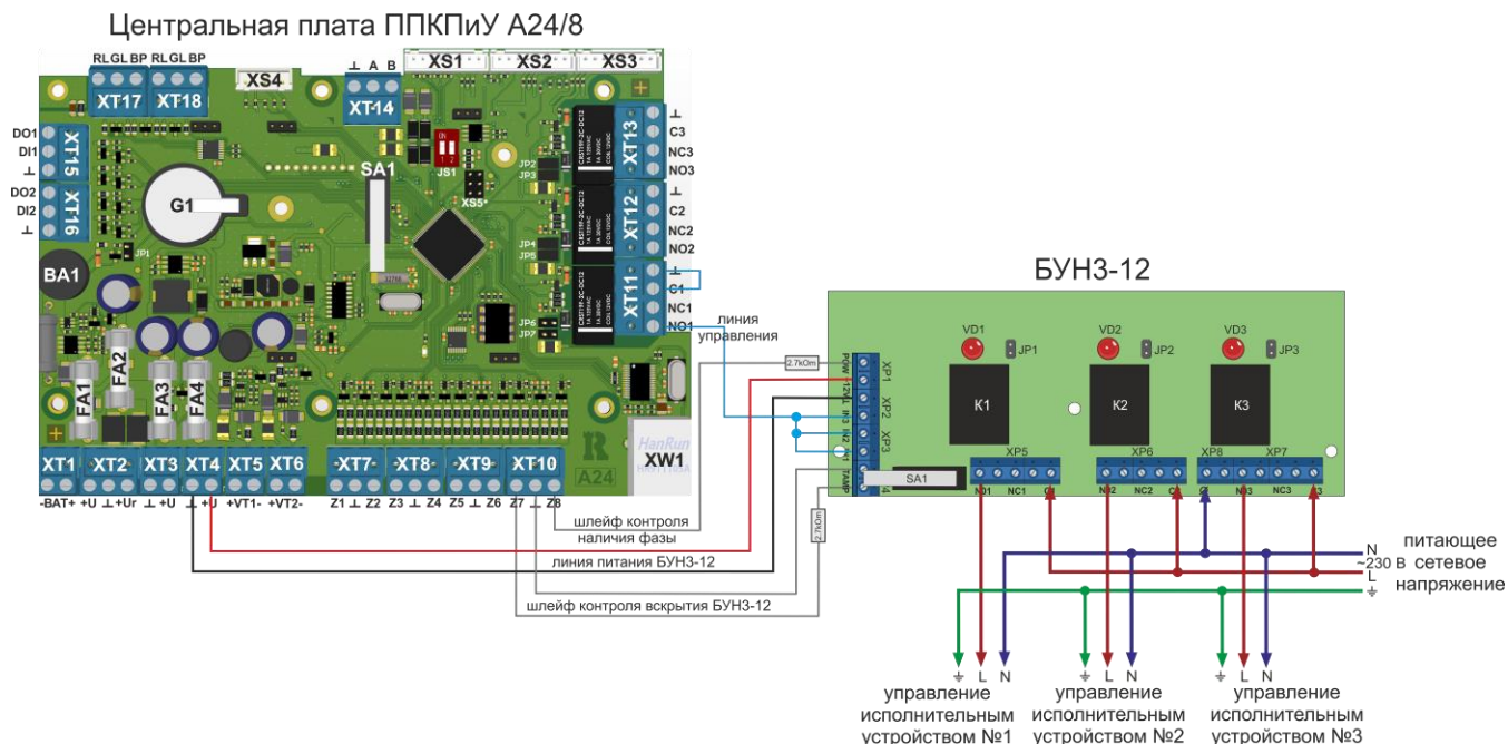
Рисунок 82. Схема подключения БУНЗ-12 к ППКПиУ А24/8.
