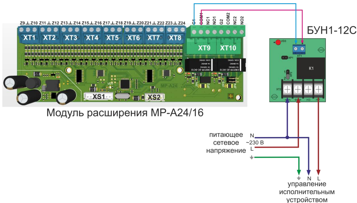
Рисунок 78. Схема подключения БУН1-12С к MP-A24/16.
