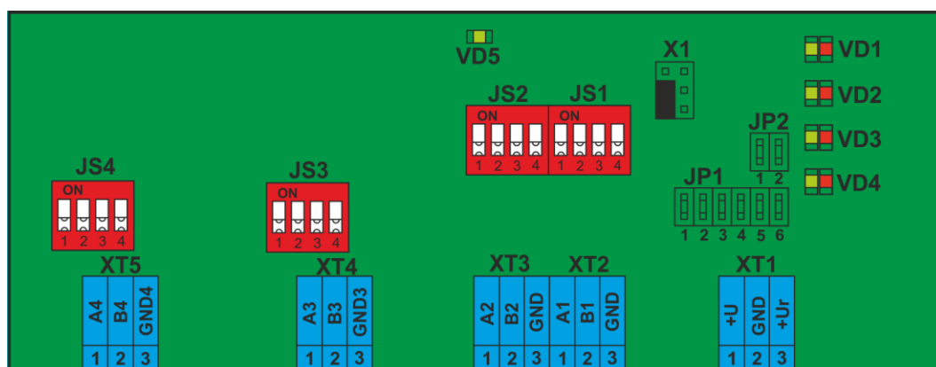
Рисунок 73. Внешний вид платы Р485
