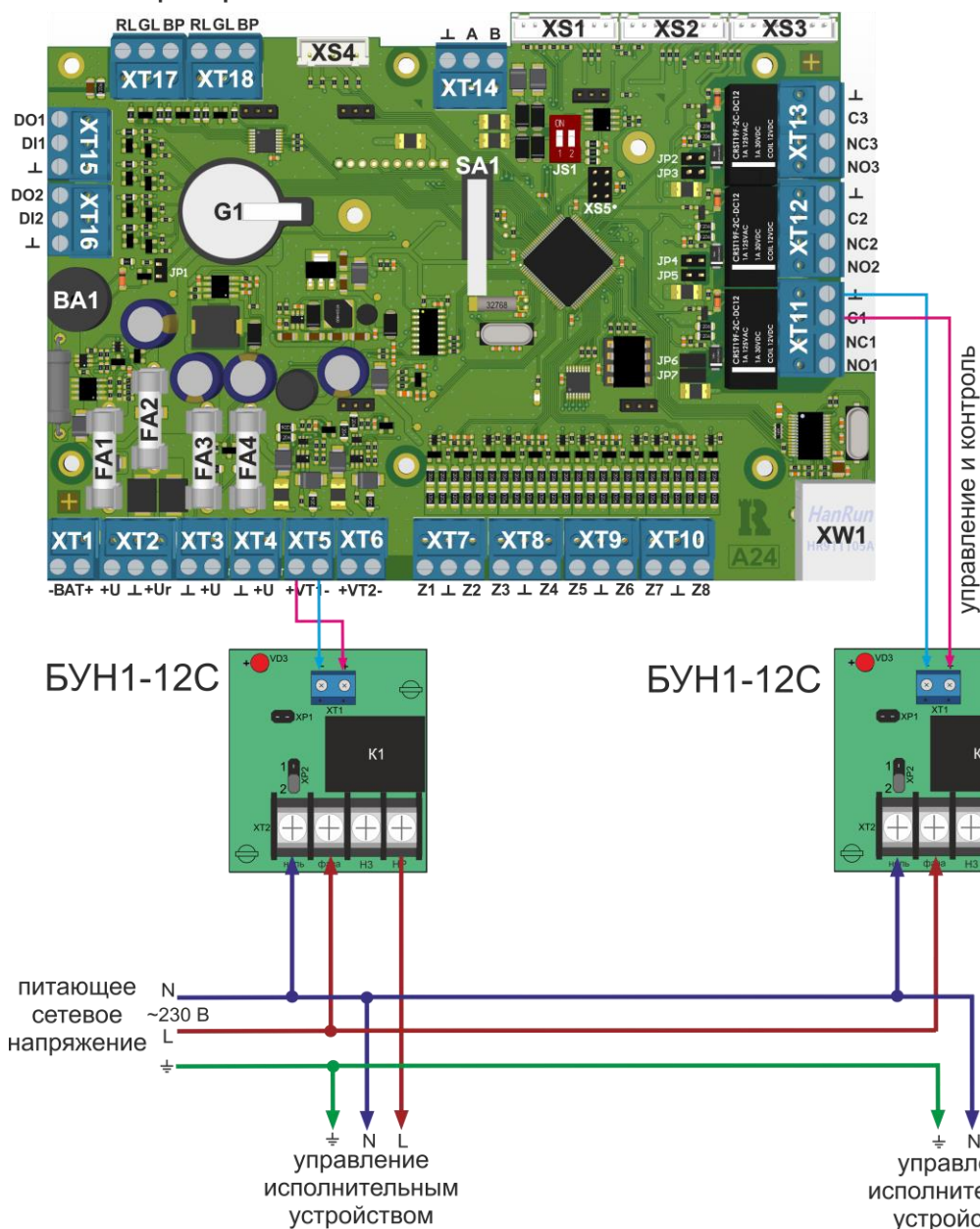
Рисунок 77. Схема подключения БУН1-12С к ППКПиУ А24/8.
