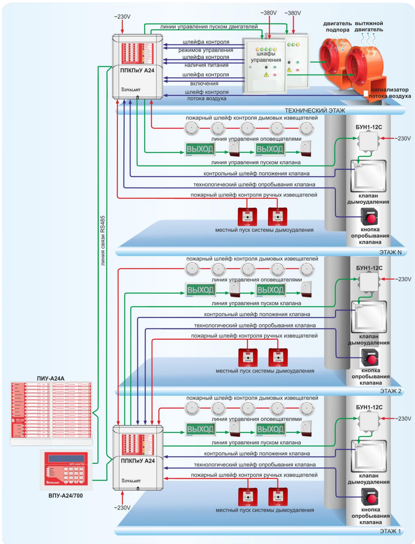
Рисунок 94. Пример структурной схемы построения систем ПС, СО и ДУ.
