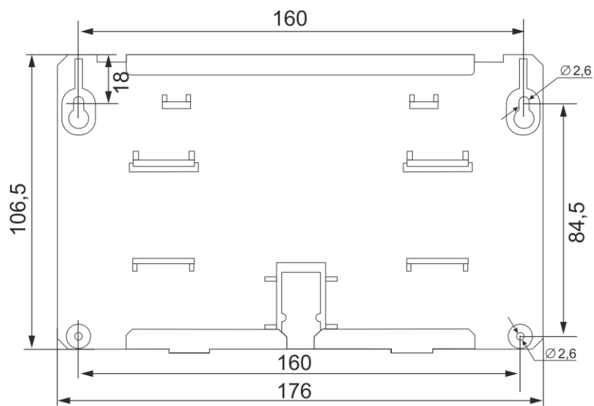
Рисунок 90. Установочный чертеж основания корпуса Р485
