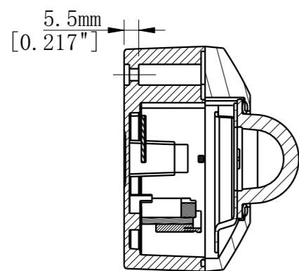
截面 A-A
