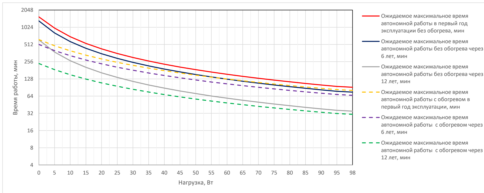
Рисунок 6.1 – график времени автономной работы шкафа Варта Бокс-4
