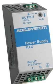
Рисунок 10.3 – промышленный блок питания на DIN-Рейку.
