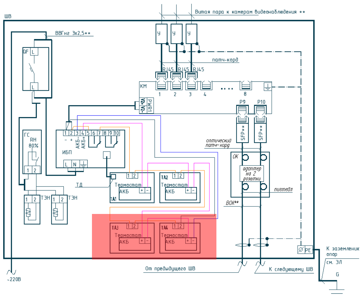
Рисунок 7.2 – схема внутренних соединений шкафа Варта Бокс
