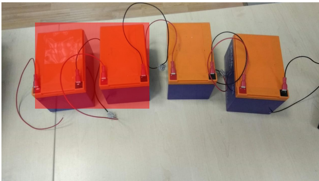
Рисунок 9.1 – подключение аккумуляторных батарей
