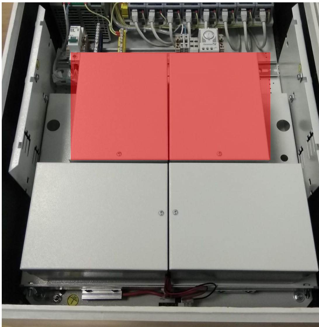
Рисунок 9.8 – Закрытые термостаты АКБ
