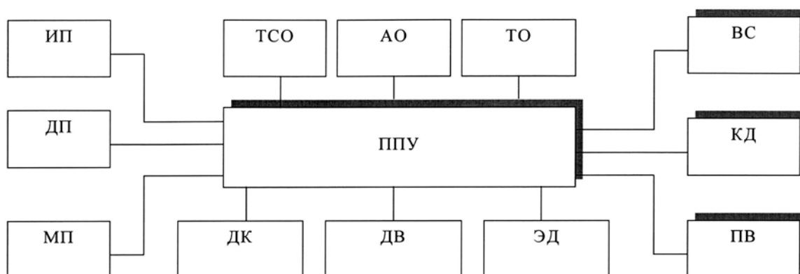
Рисунок А.3 – Схема внешних подключений ППУ установками газового, порошкового и аэрозольного пожаротушения
