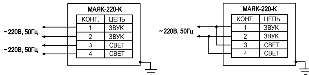
Рис. 1. Схема подключения
