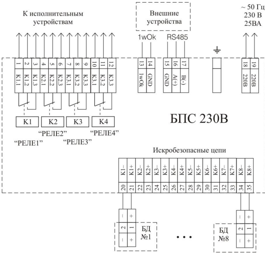
Рисунок 6.4 Монтажная схема БПС 230В.
