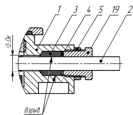
ж) открытая прокладка кабеля в кабельном вводе КВБ
