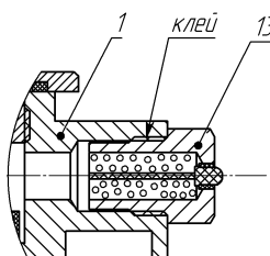
е) монтаж оконечного элемента ОЭ
