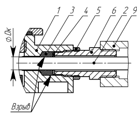
б) монтаж в трубной разводке с помощью штучера ШТ
