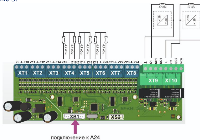
Рис. 5. Схема подключения MP-A24/16
