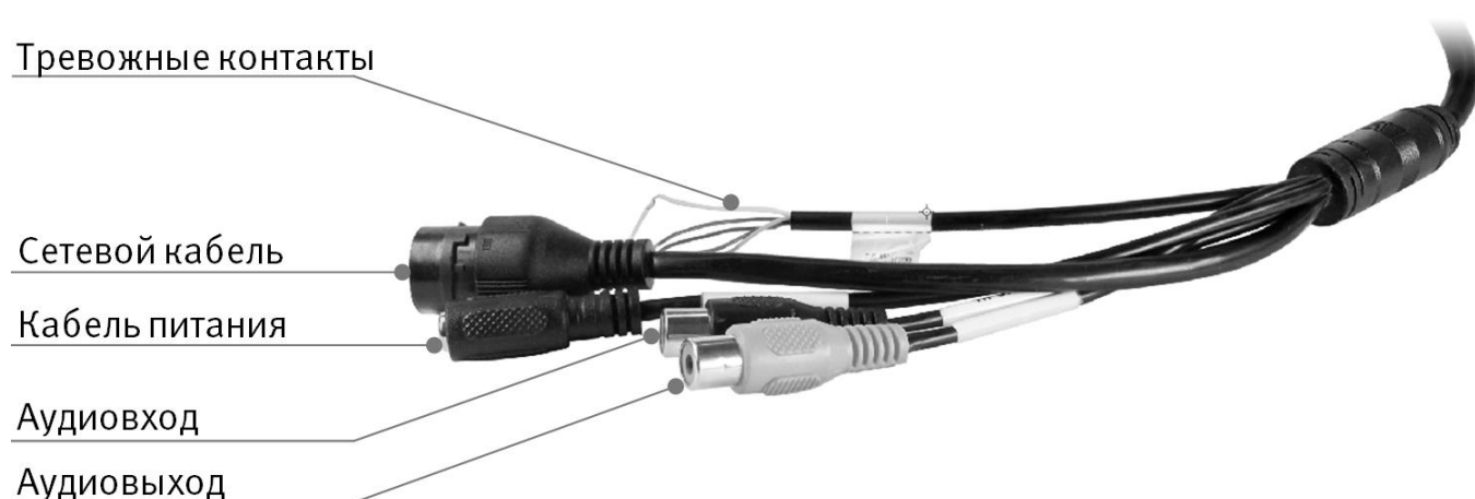
Рисунок 6.1 — Кабель видеокамеры
