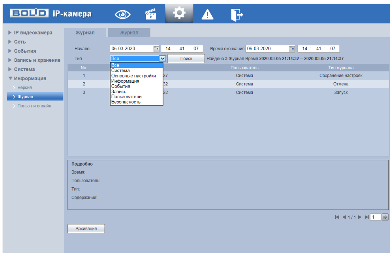
Рисунок 7.126 — Вкладка «Журнал»
