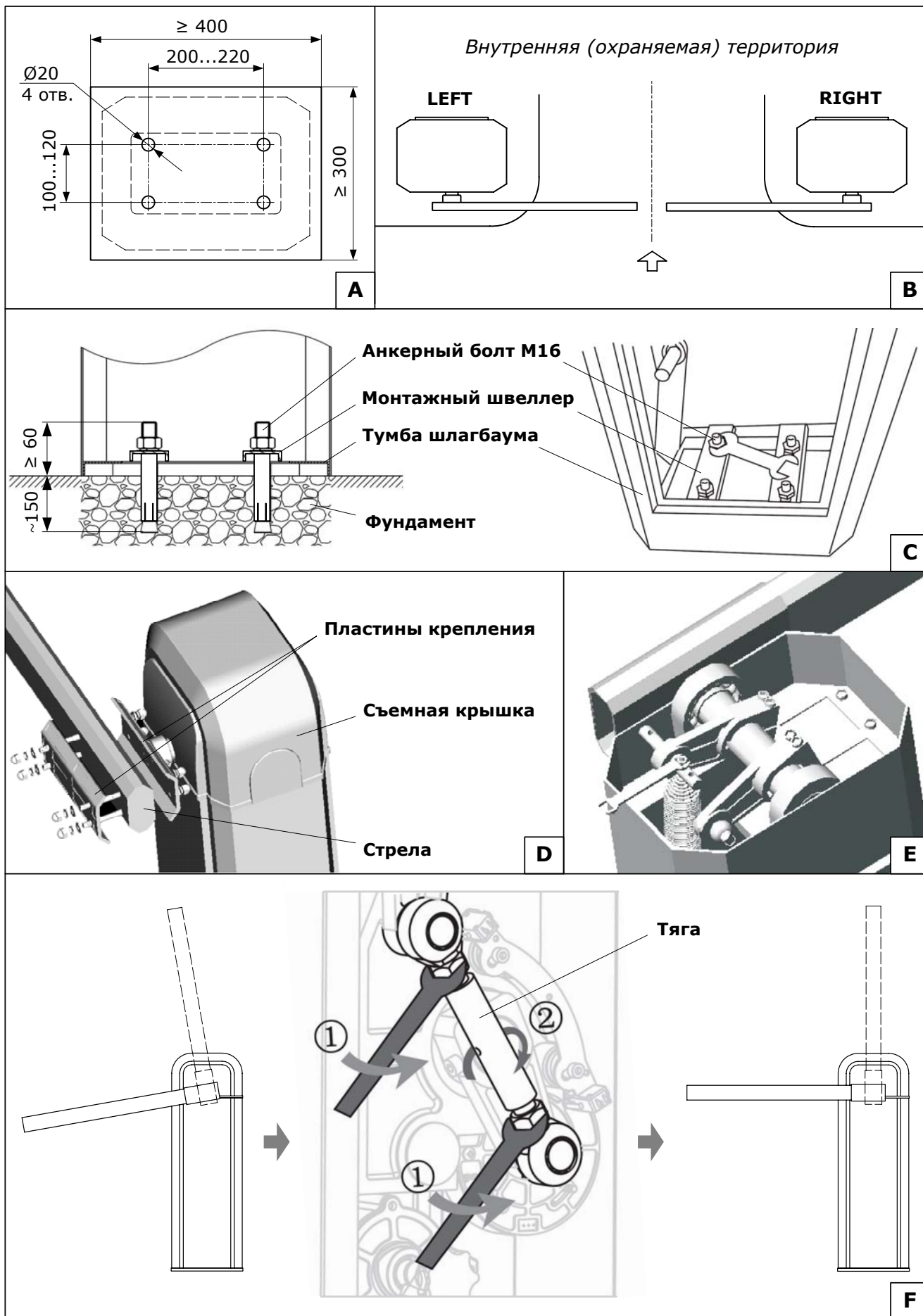
Рис. 3. Монтаж шлагбаума
