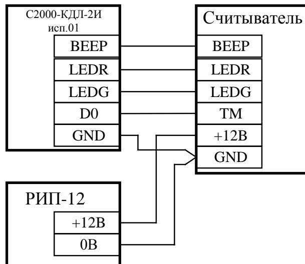
Рисунок 2.2.4.2 Схема подключения считывателей с интерфейсом Touch Memory
