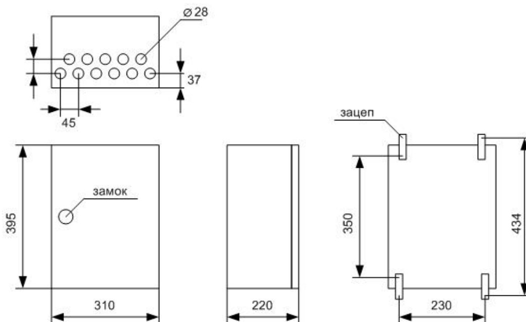
Рис. 8. Чертеж
