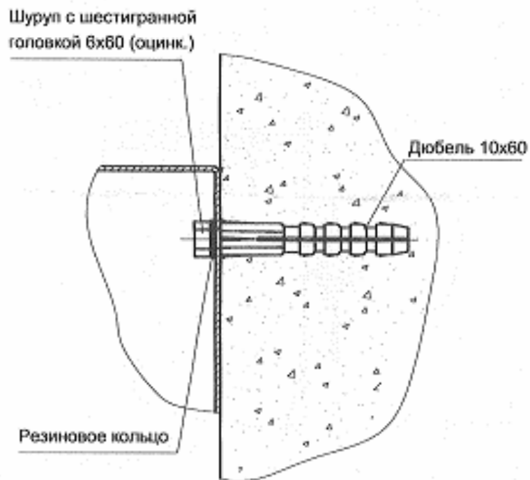
Рис. 6. Установка на стену без зацепов
