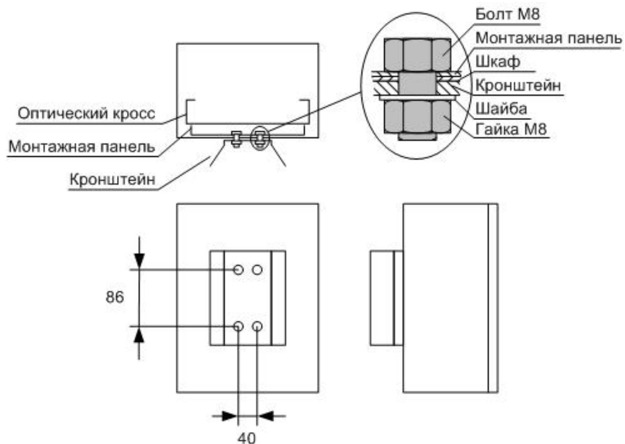
Рис. 5. Установка кронштейна для крепления шкафа на опору
