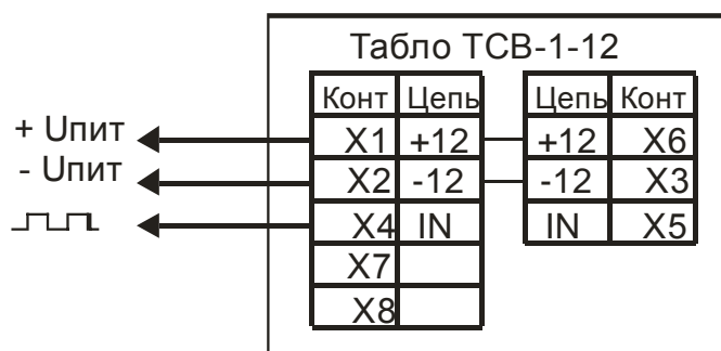
Рисунок Б.1- Схема подключения табло ТСВ-1-12, ТСВ-1Р-12, ТСВ-1Х-12 и ТСВ-1С-12 в режимах 1 и 2
