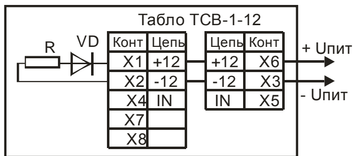
Рисунок Б.1- Схема подключения табло ТСВ-1-12, ТСВ-1Р-12, ТСВ-1Х-12 и ТСВ-1С-12 в режимах 1 и 2
