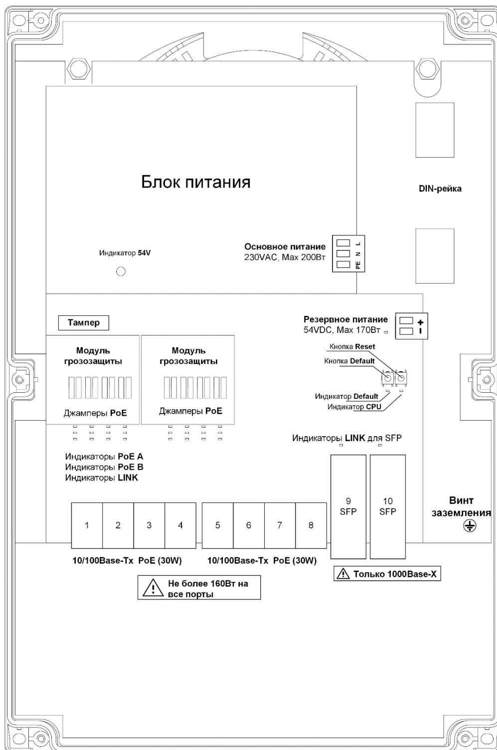
Рисунок 3.2 - Расположение элементов PSW -2G8F+
