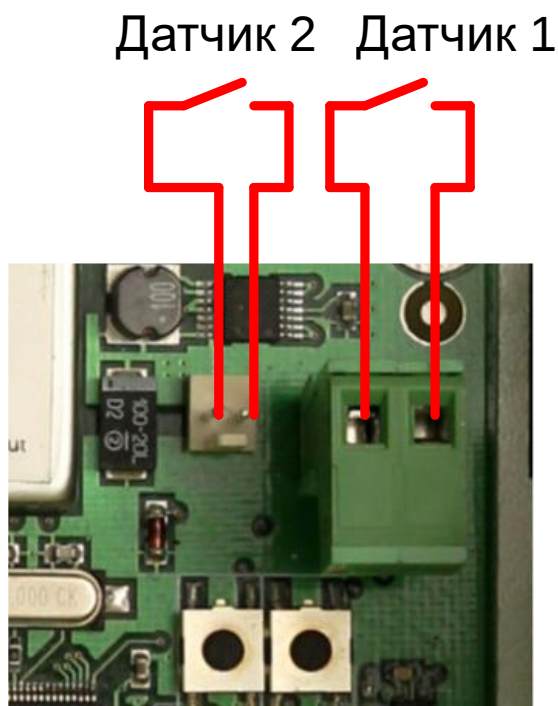
Рисунок 3.6 - Сухие контакты
