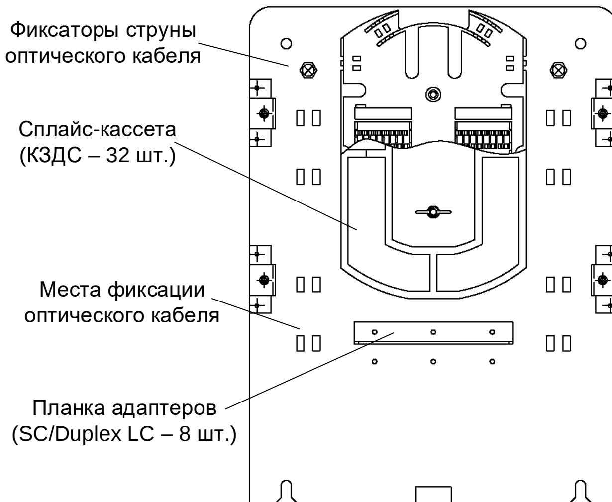
Рисунок 3.4 - Оптический кросс
