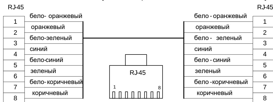
Рисунок 7.4 - Разделка кабеля.
