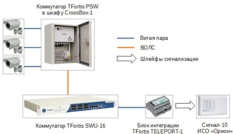
Рис. 5.3.27.1 Структура сети
