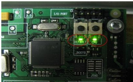
Рис.1.1. Индикаторы DEFAULT и CPU – коммутаторы PSW
