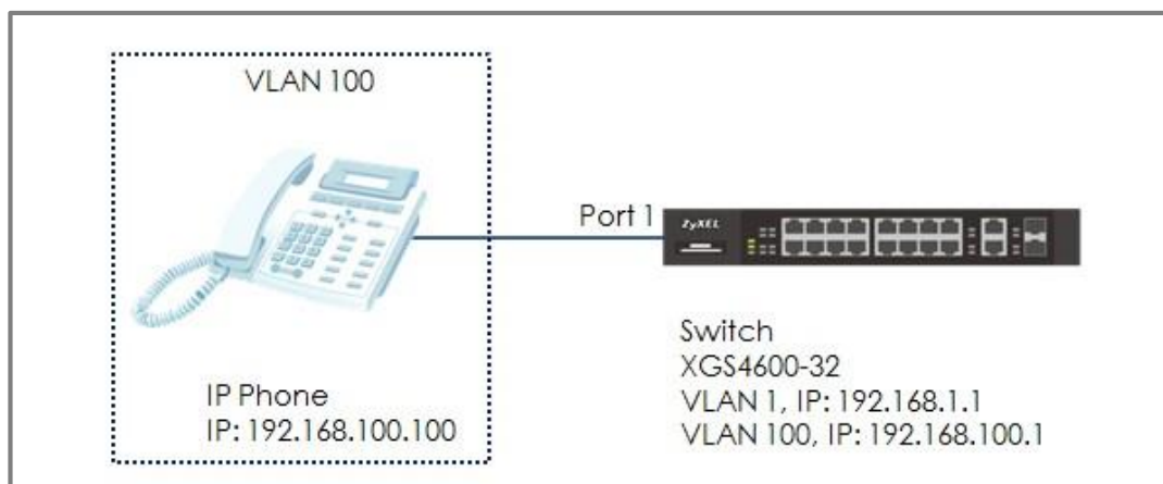
Иллюстрация 23 Использование LLDP-MED для настройки VLAN для IP-телефона
