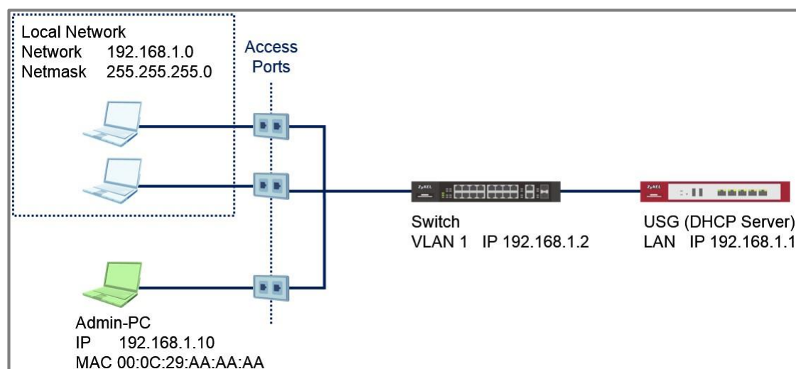
Иллюстрация 27 У устройства, используемого администратором и подключенного к порту доступа, статичный IP-адрес
