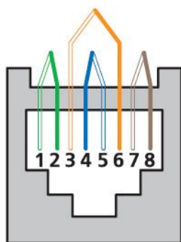
Раскладка проводников в соответствии с TIA/EIA 568A
