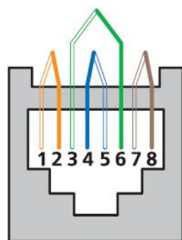
Раскладка проводников в соответствии с TIA/EIA 568B
